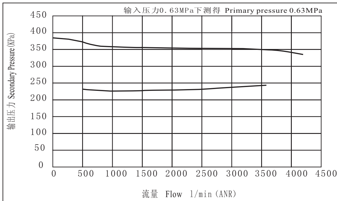
流量特性曲线 Flow characteristics
