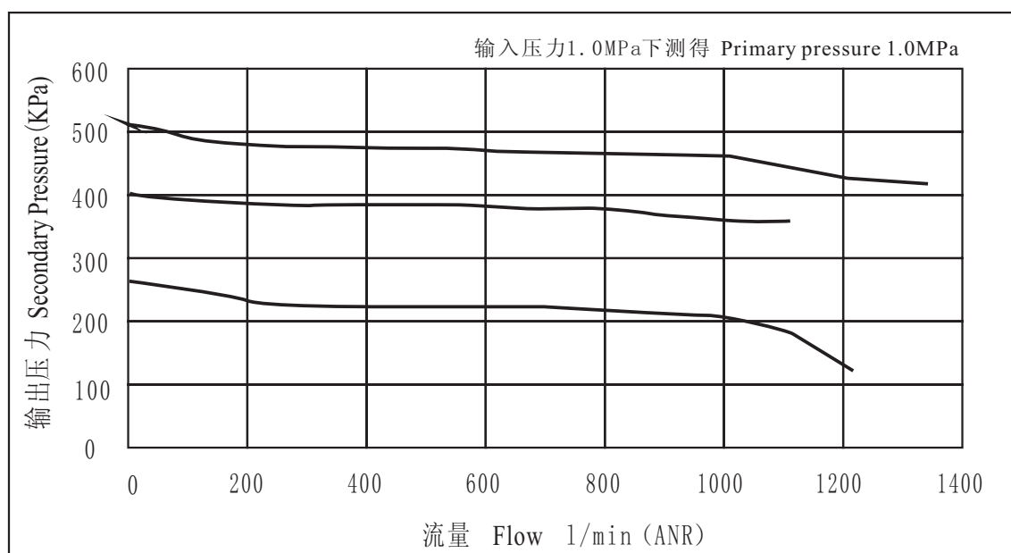
流量特性曲线 Flow characteristics
